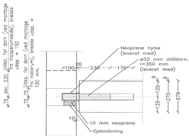
Detalje ved dornsamling (1:10)
